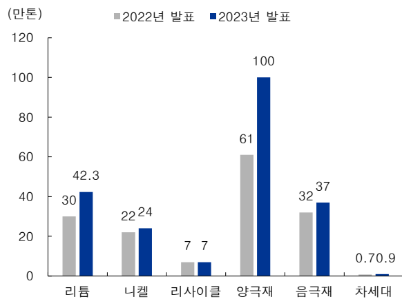
그림 144. 2030년 기준 2차전지 소재 CAPA 상황
