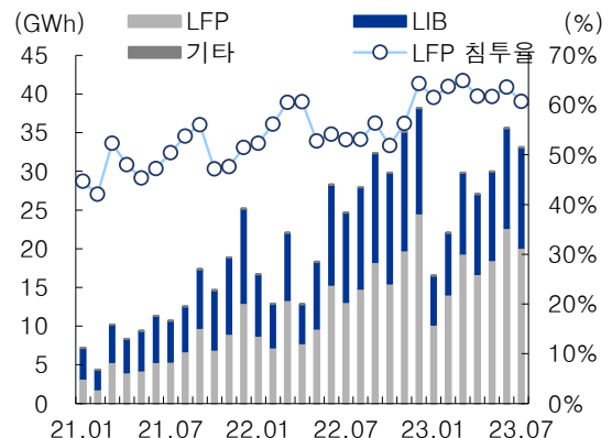
그림 112. LFP 배터리 침투율 추이(중국)
